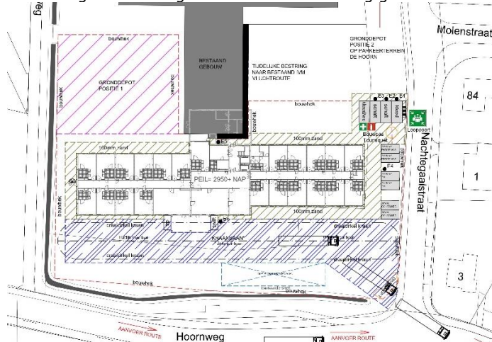
Afbeelding 4: inrichting bouwterrein rond huidige gebouw
